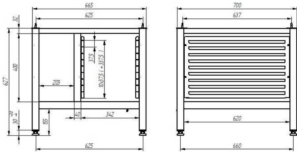
rys 2. Wymiary podstawy pod piec 000.T-PK10
