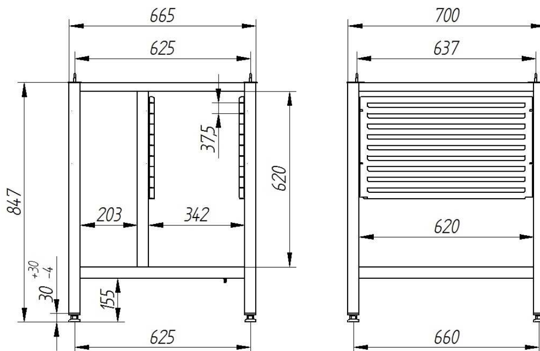
rys 1. Wymiary podstawy pod piec 000.T-PK
